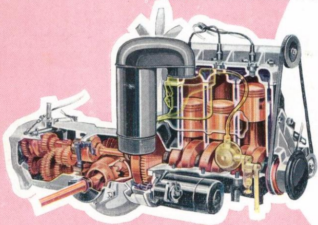
Schnittbild des bewährten DKW-Zweitakt-Freud
