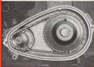
Kraftübertragung vom Motor zum Getriebe und die geschützte Abdichtung des Kettenkastens
