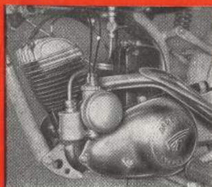
Motor und Getriebe bilden eine Einheit. Der Kettenkasten hat nur zwei Klemmschrauben!
